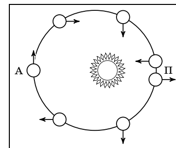
Рис. 15. Резонанс между суточным и орбитальным вращением Меркурия. Показаны различные положения планеты на орбите; стрелка указывает ориентацию одного из полушарий Меркурия.
